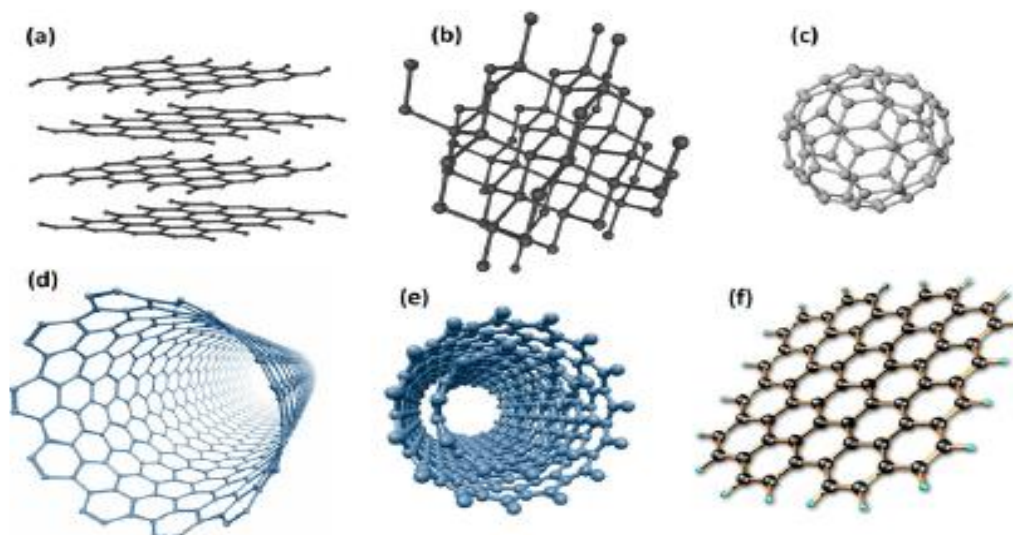
Figura 18. Diferentes dimensões observadas na estrutura do carbono: a) Grafite(3D); b) Diamante(3D); c) Fulereo(0D); d) Nanotubos de carbono de parede única(1D); e) Nanotubos de paredes múltiplas(1D); e f) Grafeno(2D)
