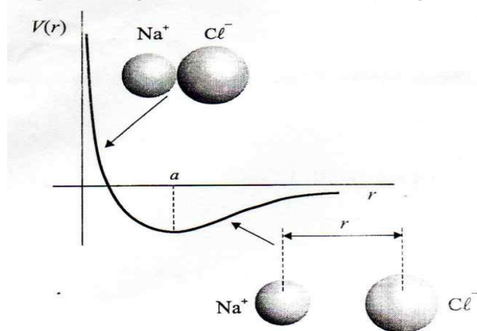
Figura 6. A energia de interação efetiva entre o \text{Na}^+ e \text{Cl}^- em função da distância
