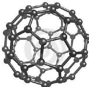
Figura 20. Fulereo C 60
