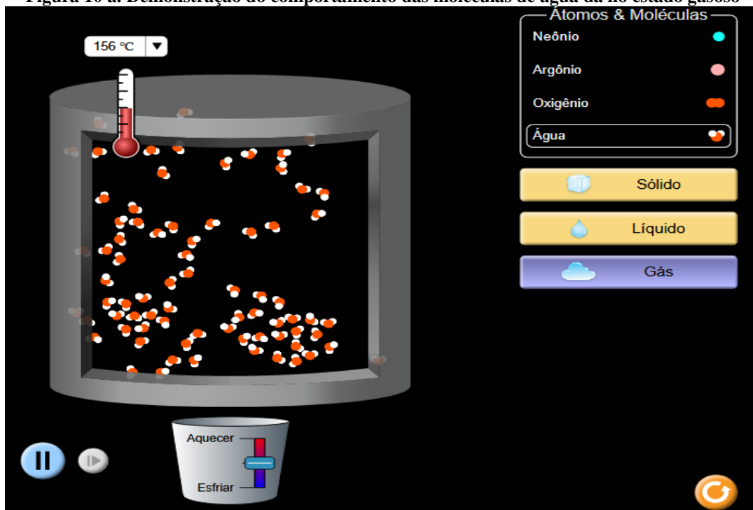
Figura 10 a. Demonstração do comportamento das moléculas de água da no estado gasoso
