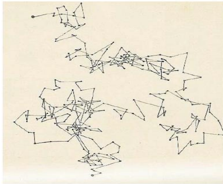
Figura 10. Partícula executando o movimento Browniano
