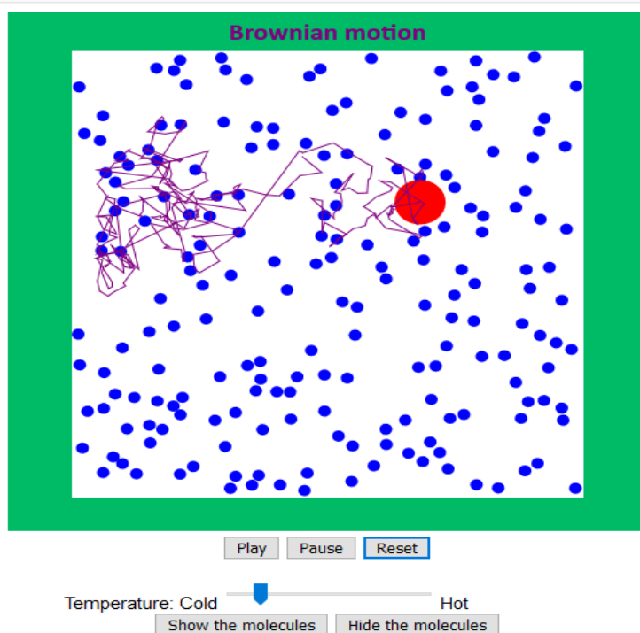
Figura 16 a. Simulação do movimento Browniano
