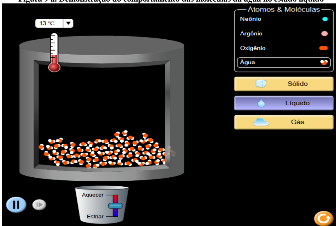
Figura 9 a. Demonstração do comportamento das moléculas da água no estado líquido
