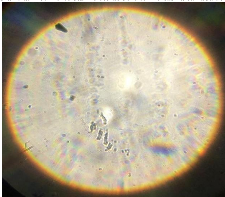
Figura 15 a. Movimento das moléculas de leite imersas na camada de água
