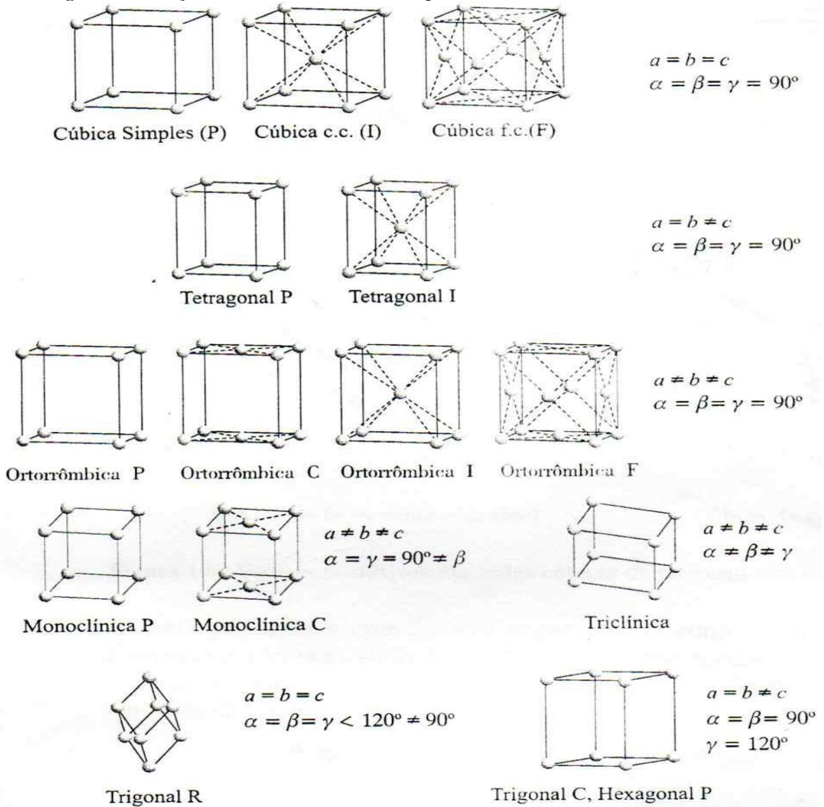
Figura 9. Ilustração das células unitárias das 14 possíveis redes cristalinas em três dimensões.
