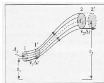
Figura 1.9 – Filete de corrente de um fluido ideal em um escoamento estacionário.
