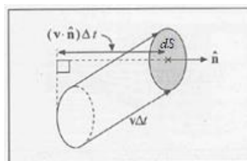
Figura 1.8 – Massa que atravessa dS e normal externa \hat{n} .
