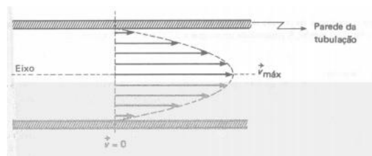
Figura 1.12 – Perfil parabólico da velocidade de um fluido. (Fonte: NUSSENZVEIG, H. M., vol. 2, 2002, p. 34)
