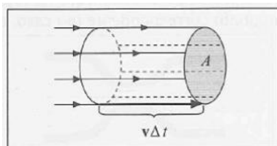
Figura 1.6 – Massa do fluido que atravessa a seção A com velocidade do fluido em um instante \Delta t .
