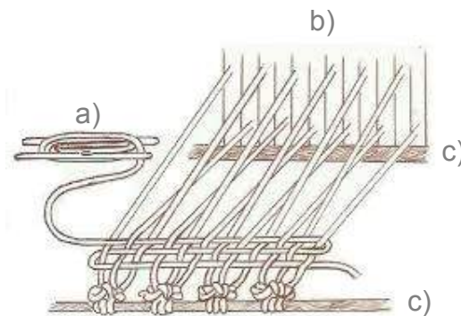
Fig. 34 – Representação gráfica do processo fabril da estrutura do tecido.
